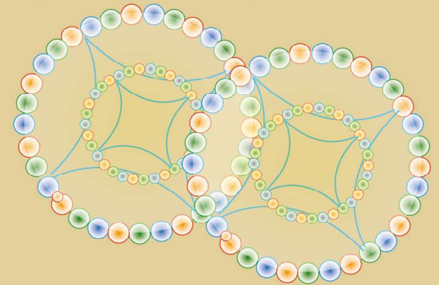
Cells - Pervading
